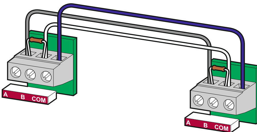
Rys. 12. Przykład magistrali komunikacyjnej łączącej centralę i panel wyniesiony.
